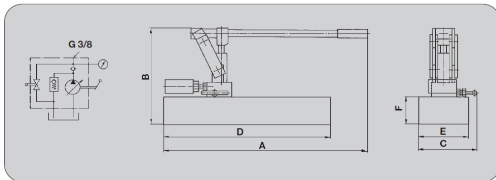
Darstellung von einfachwirkender Handpumpe
